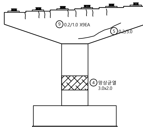
배면
